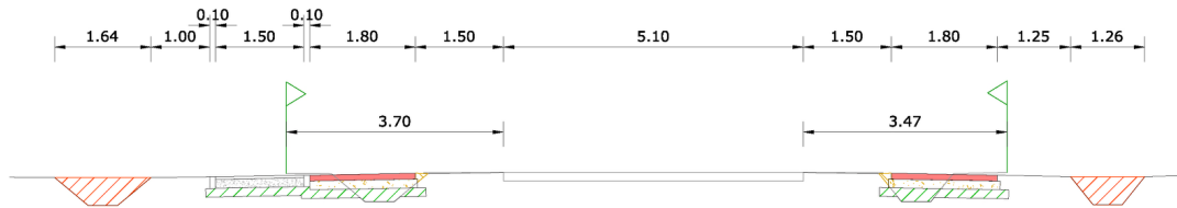
dwarsprofiel A-A
