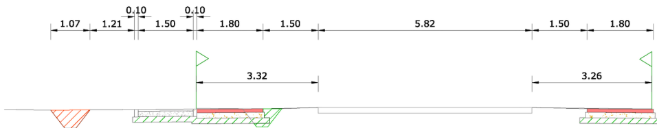
dwarsprofiel C-C
