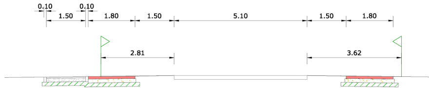
dwarsprofiel B-B
